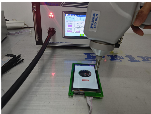
图 5-2 ESD 测试图
